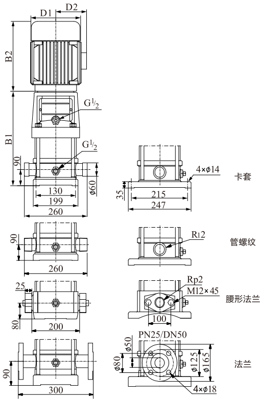
安装图
