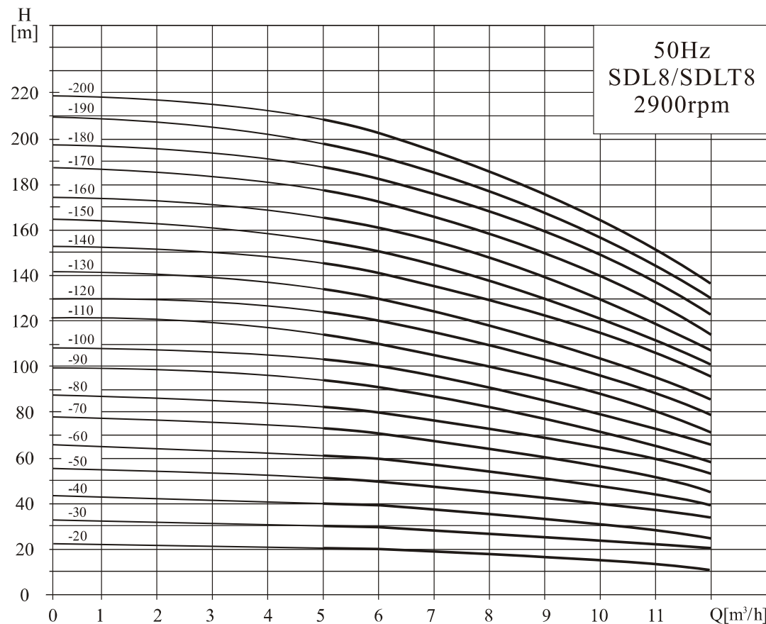
性能曲线
