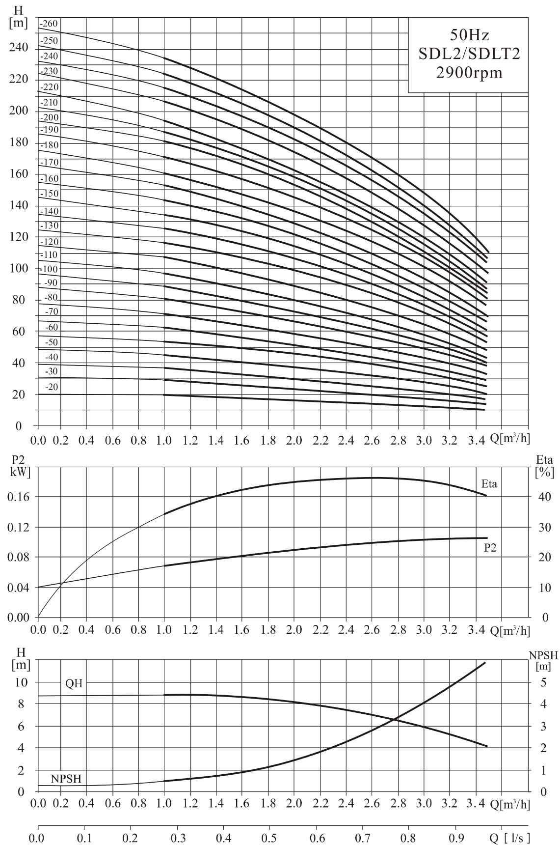
性能曲线
