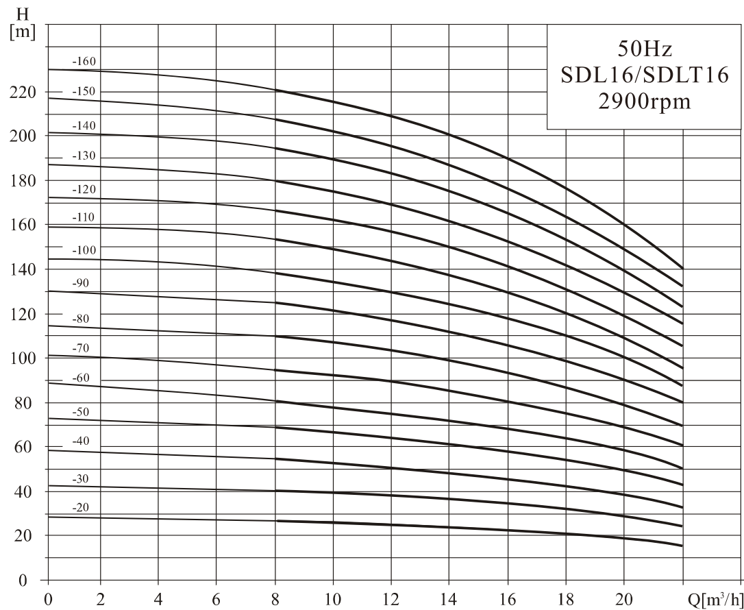
性能曲线
