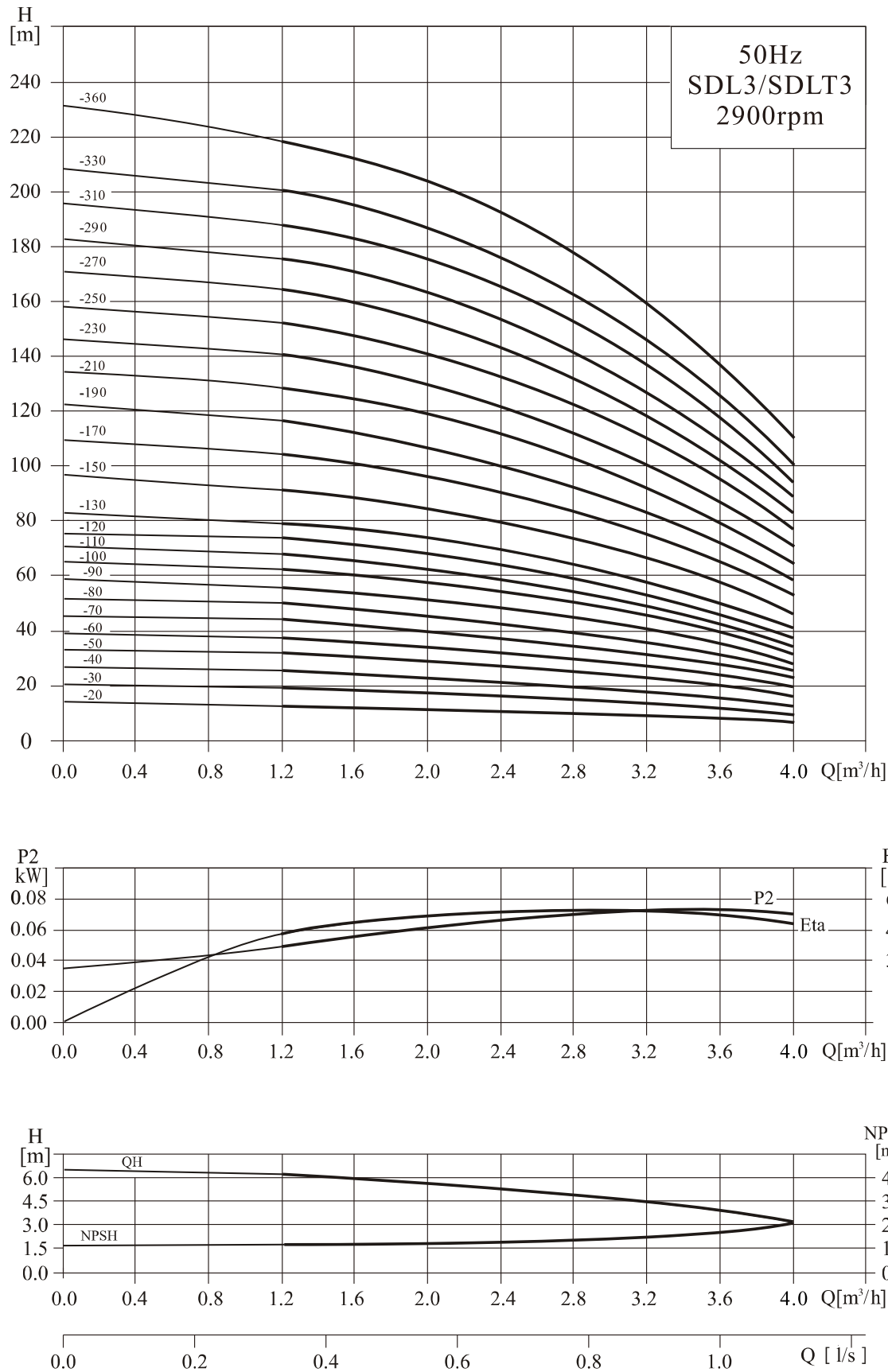
性能曲线
