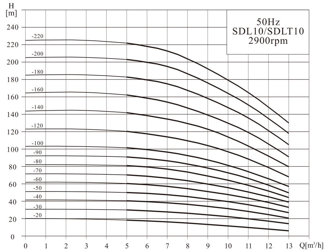
性能曲线
