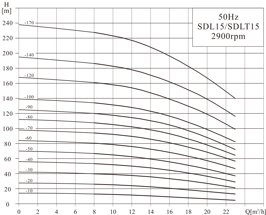
性能曲线
