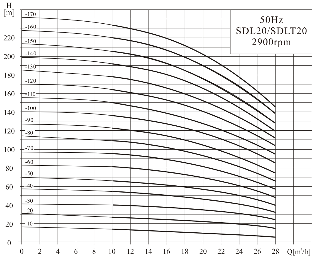
性能曲线
