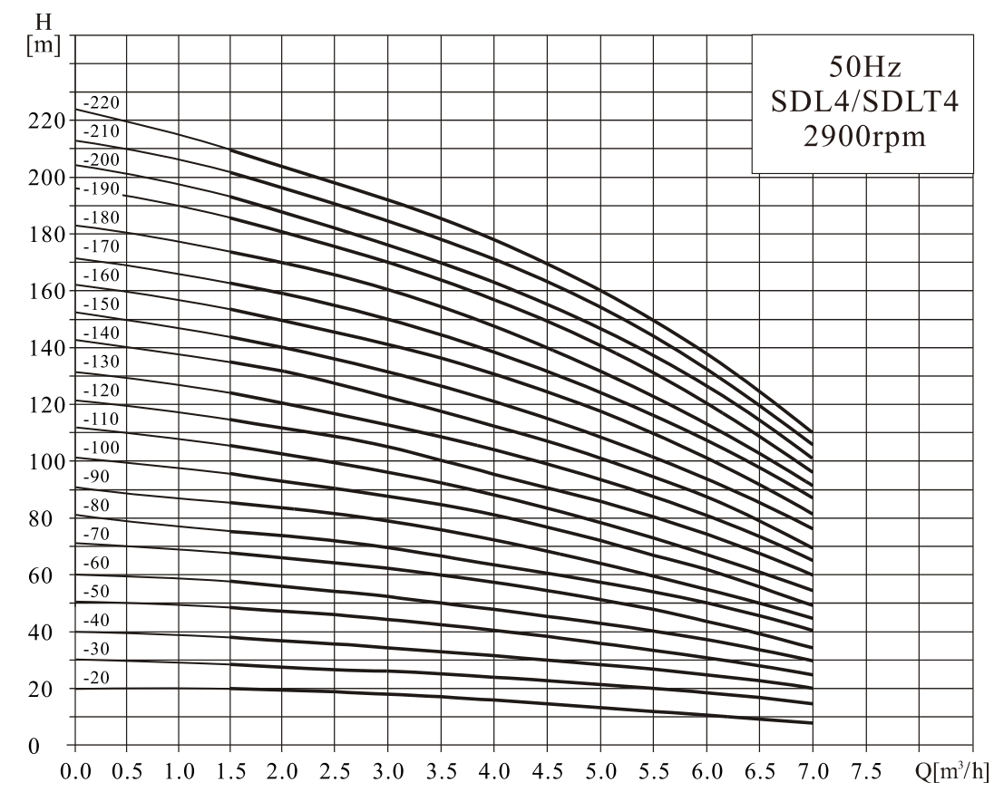
性能曲线
