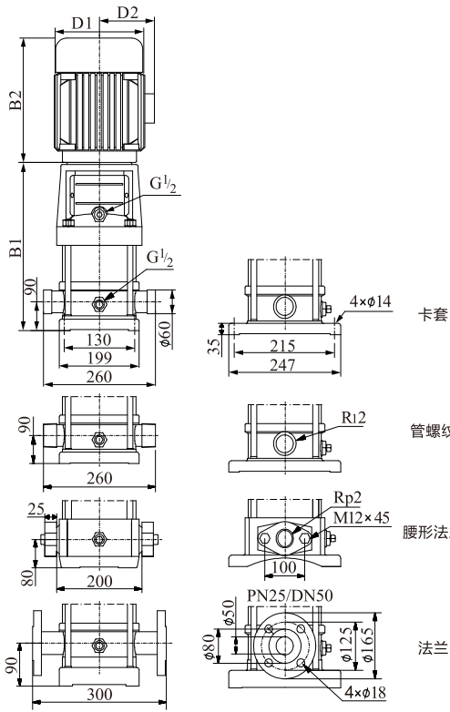
安装图
