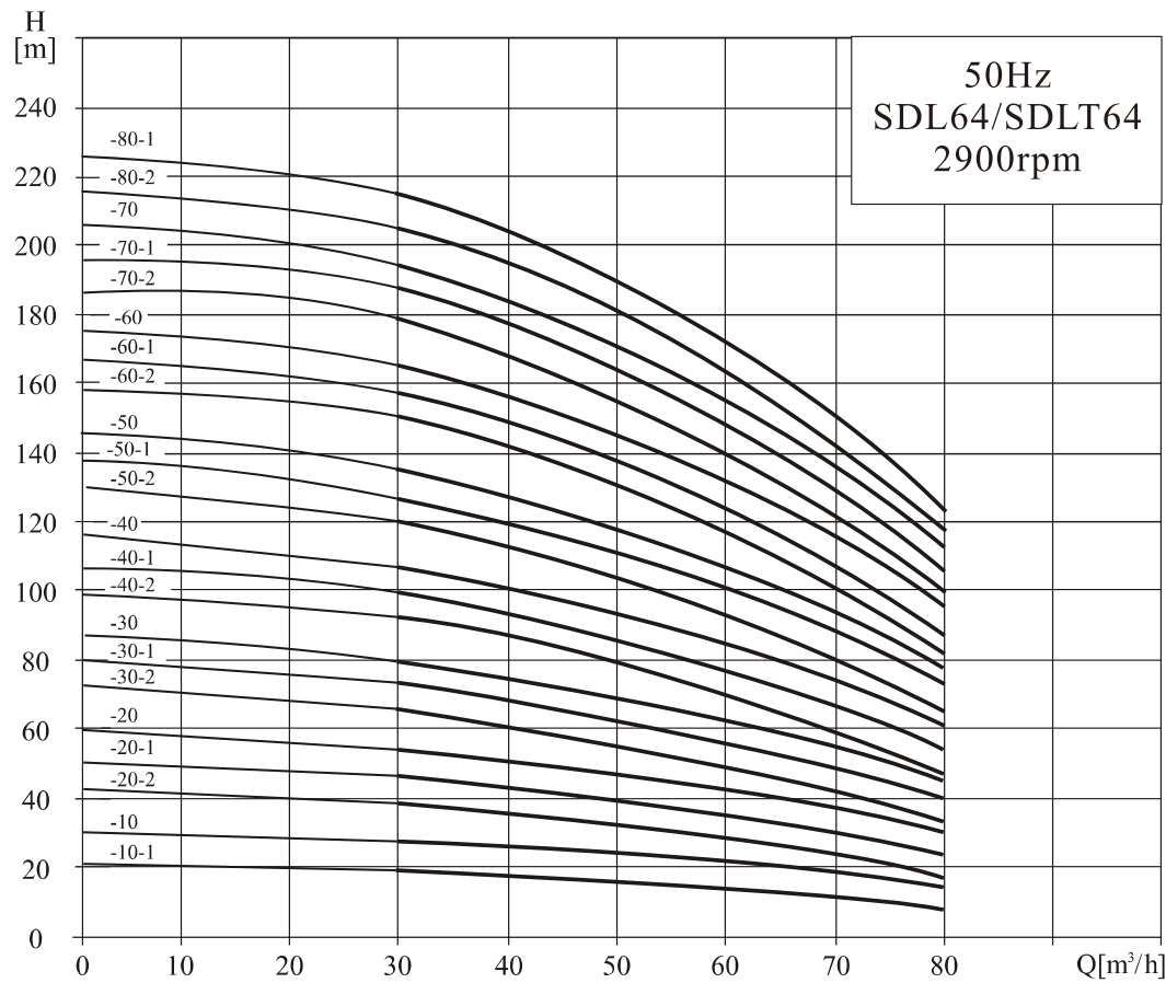
性能曲线
