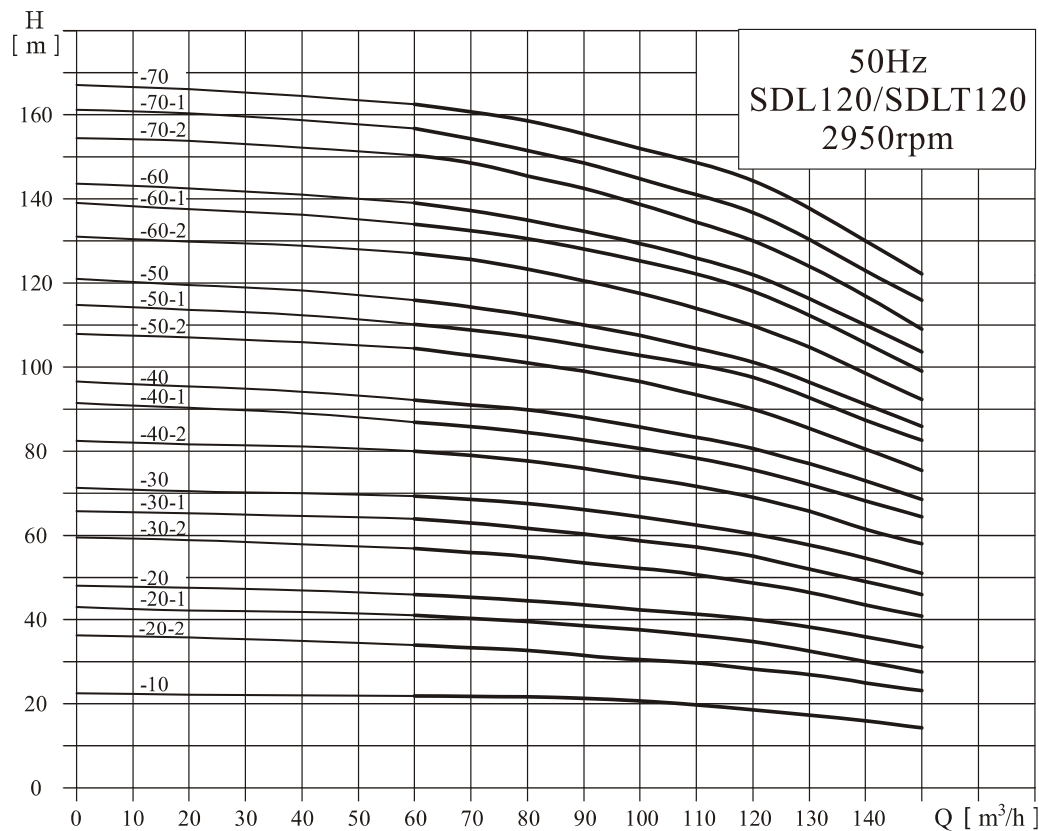
性能曲线
