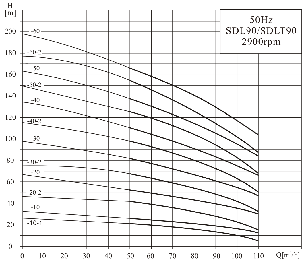
性能曲线
