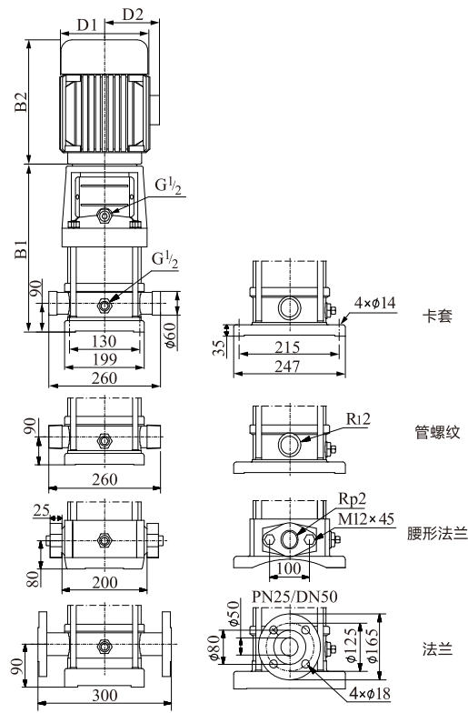
安装图
