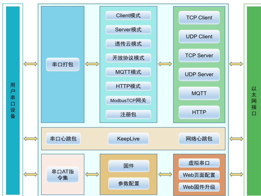
HP-E10功能框架示意图
