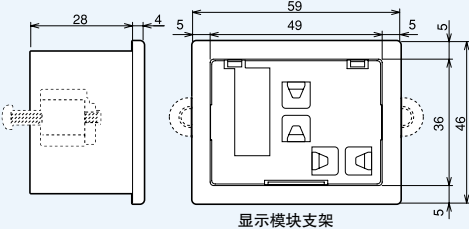
FX3U-7DM-HLD
