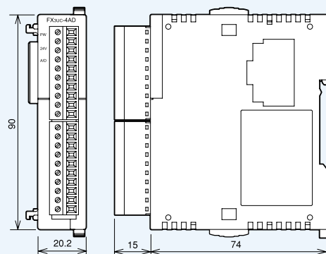
FX3UC-4AD
