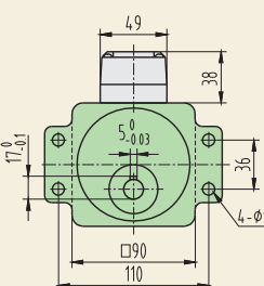
带耳减速箱
