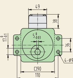
带耳减速箱
