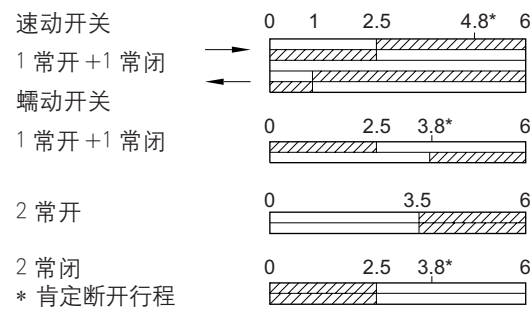
开关行程图
