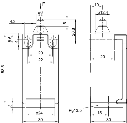
产品外观及外形尺寸
