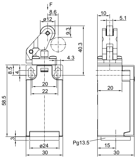
产品外观及外形尺寸
