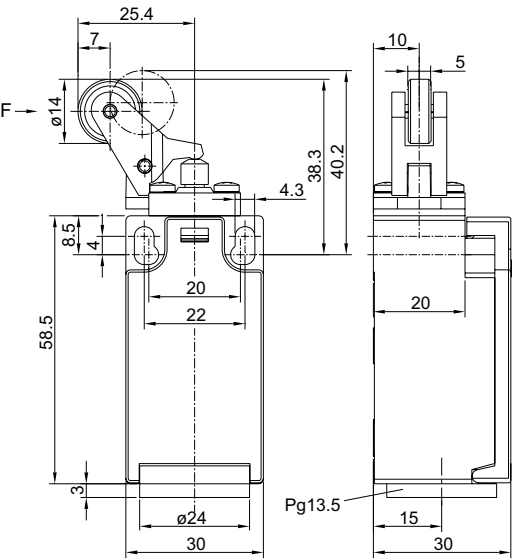
产品外观及外形尺寸
