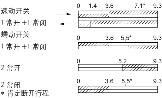
开关行程图
