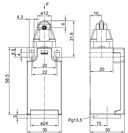
产品外观及外形尺寸
