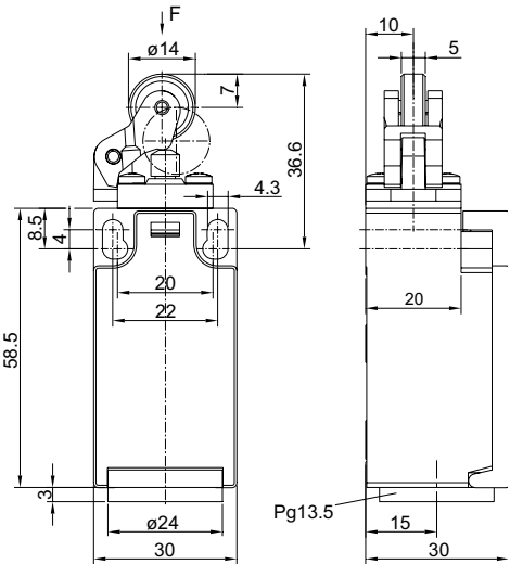
产品外观及外形尺寸
