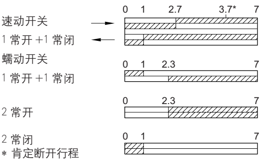
开关行程图
