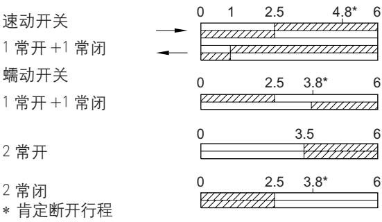
开关行程图
