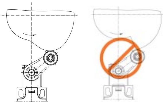
凸轮的下降边缘
